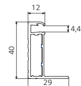
Frame Dwarsdoorsnede
